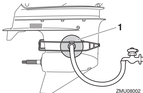
1. Spülaufsatz
