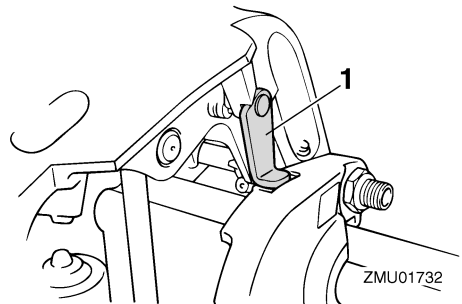
1. Ankippr-Arretierungshebel
