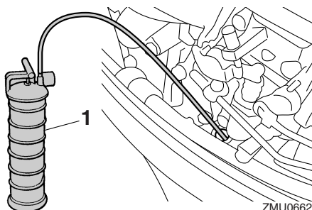
1. Ölwechsler
